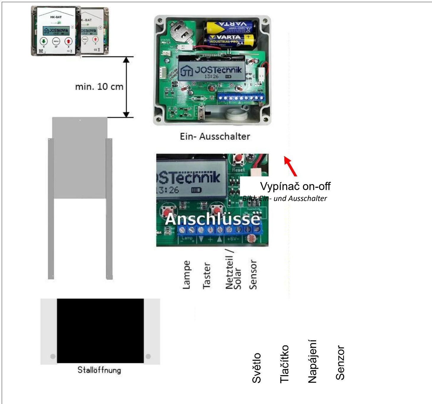
Obrázek: montáž samostatného zařízení
